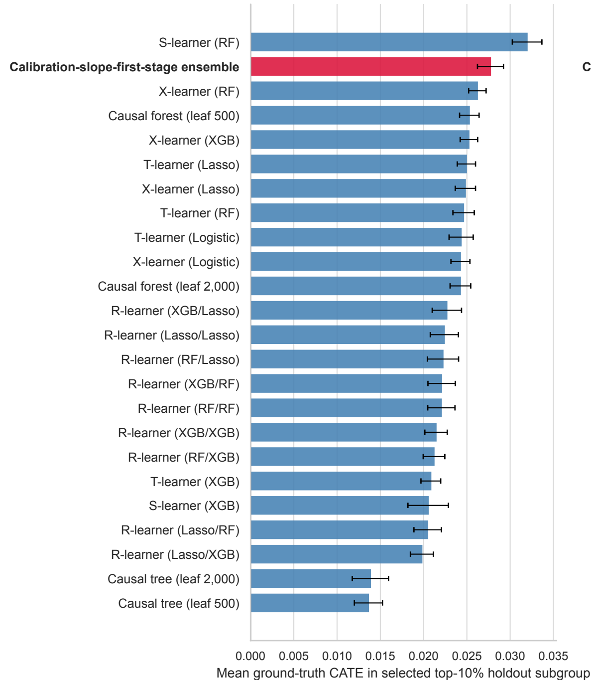
DGP1
