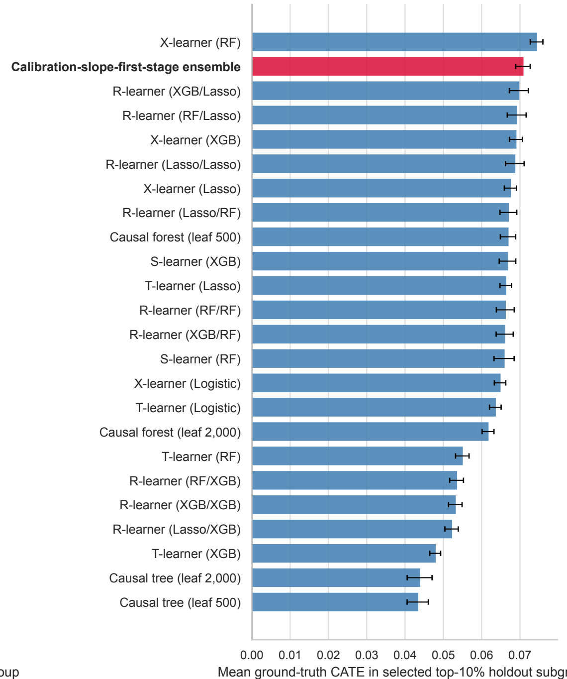
DGP2
